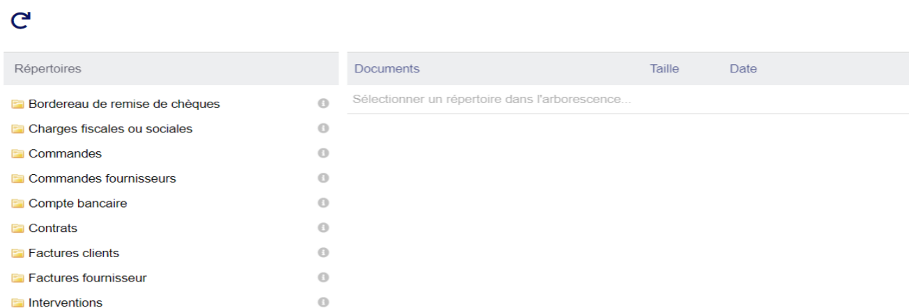
Figure 14.24 – Répertoires automatiques
